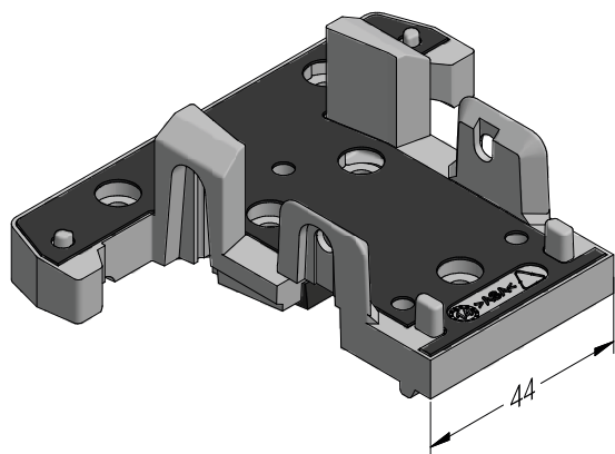
Держатель порога импоста 96 SYNEGO®
