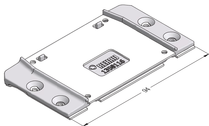
Механический соединитель импоста 124 AD SYNEGO® литой металлический
