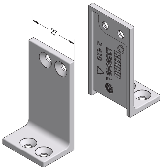
Набор уголков для крестовых соединений импоста MD SYNEGO® литой металлический
