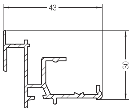
Добавочный профиль SYNEGO®
