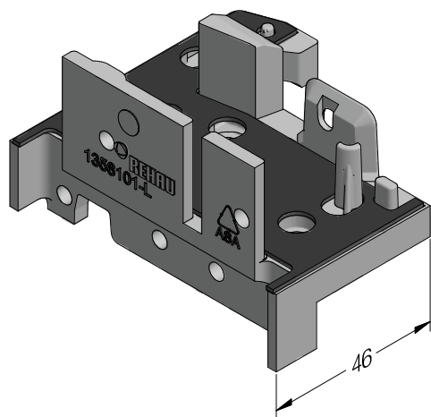
Держатель порога коробки 72 SYNEGO®
