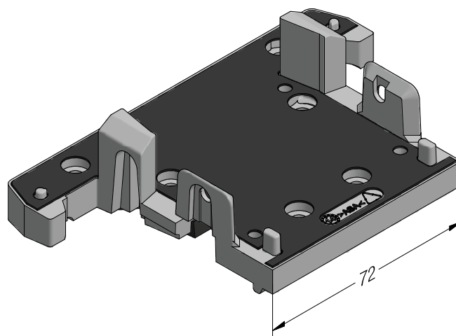
Держатель порога импоста 124 SYNEGO®
