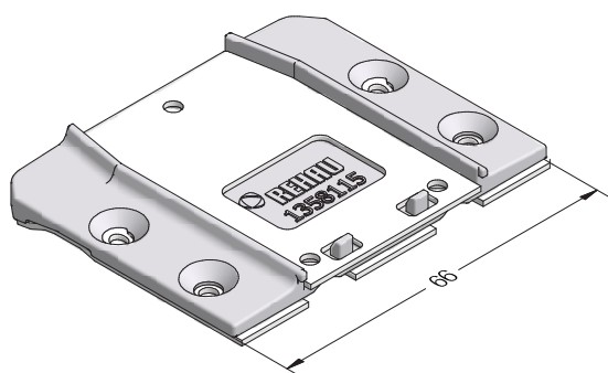
Механический соединитель импоста 96 AD SYNEGO® литой металлический
