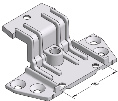
Механический соединитель импоста 96 MD SYNEGO® для крестовых соединений
