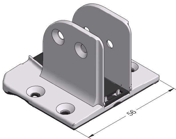
Механический соединитель горбылька 68 SYNEGO® литой металлический
