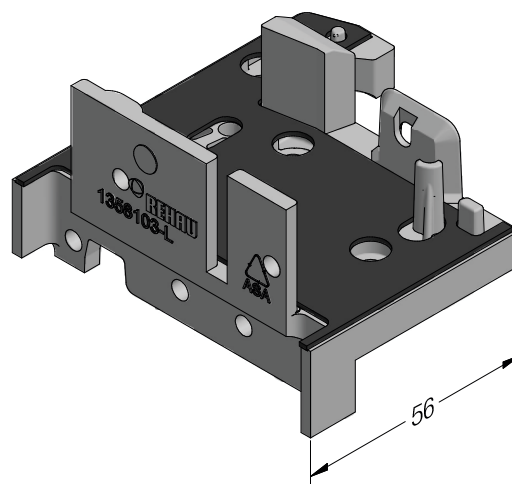
Держатель порога коробки 82 SYNEGO®
