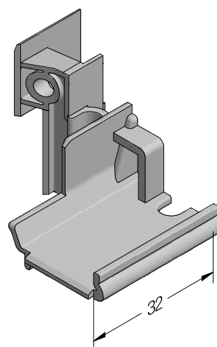
Торцевой колпачок добавочного профиля SYNEGO®
