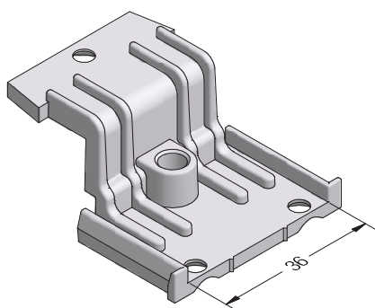
Механический соединитель импоста 96 MD SYNEGO® литой металлический
