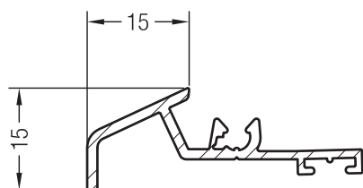
Слезник 15 BT70
