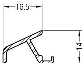
Слезник 14 BT70
