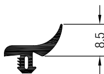
Уплотнение дверное №2 (для дверной створки T)
