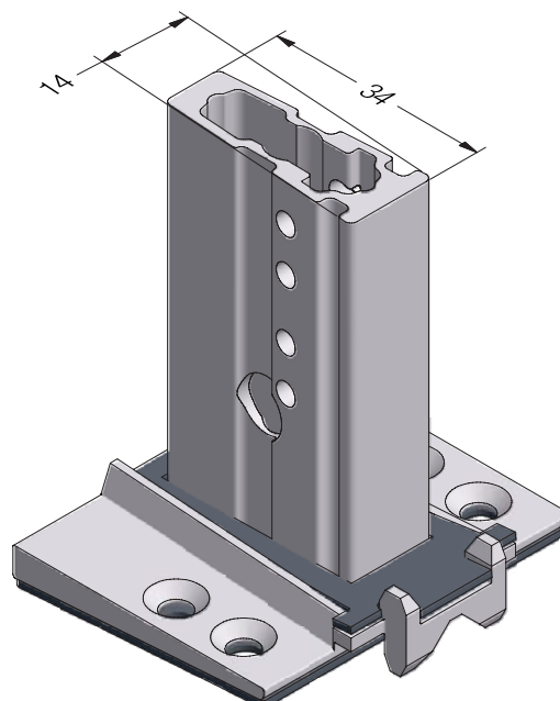
Механический соединитель ZDG горбылька 68 BT70
