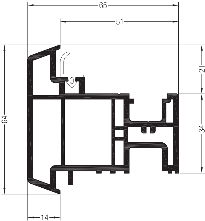
Ложный импост №1 BT70 (в комбинации со створкой входной двери Z)
