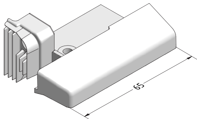
Торцевой колпачек слезника 15 шульповой створки BT70 ASA
