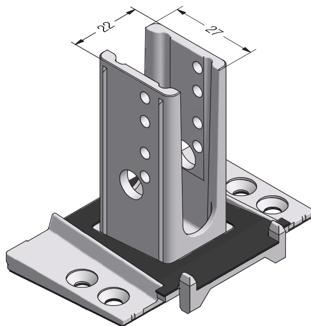
Механический соединитель ZDG для импоста 86 BT70
