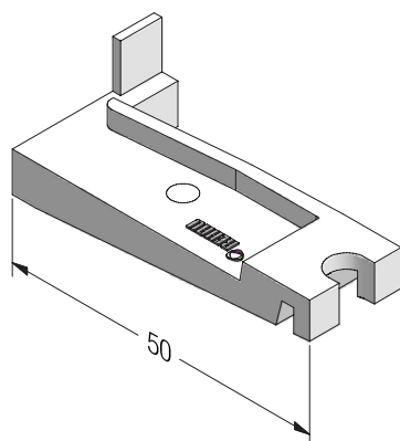
Торцевой колпачок порога RAU-TPE
