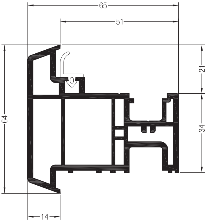
Ложный импост №1 BT70 (в комбинации со створкой входной двери T)
