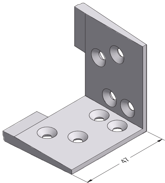
Уголок для установки горбылька или импоста в коробку BT70 Литой металлический
