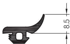
Уплотнение дверное №1 (для дверной створки Z)
