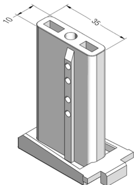
Механический соединитель горбылька 68 BT70
