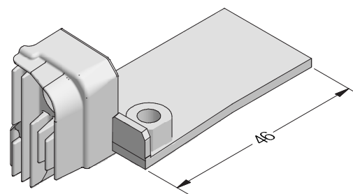
Торцевой колпачек слезника 15 шульповой внешней створки BT70 ASA
