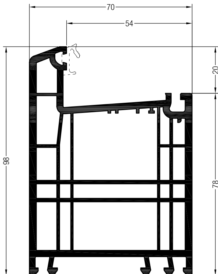
Профили коробок
