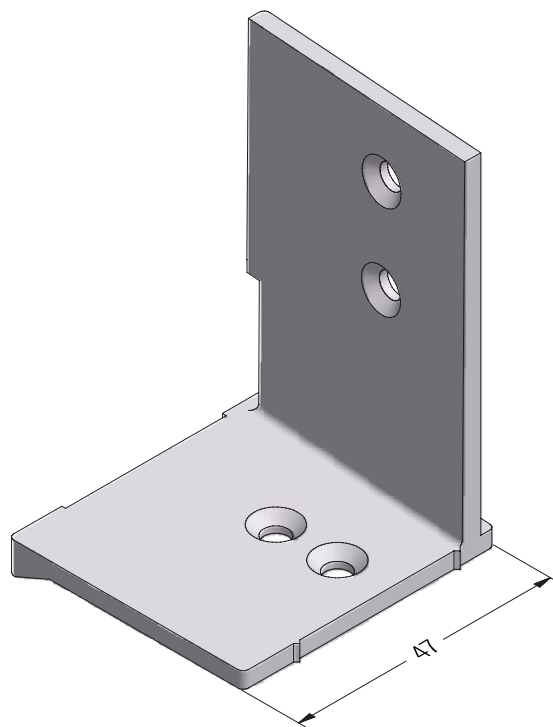
Уголок для установки горбылька или импоста в створку 48 круглую BrID. Литой металлический
