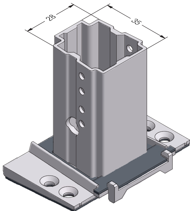
Механический соединитель ZDG для импоста 86 BT70
