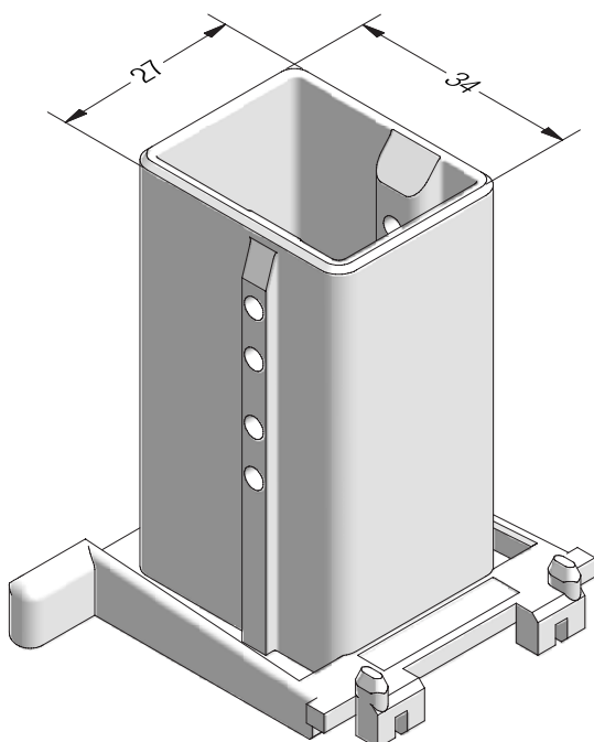
Механический соединитель №1 для импоста 86 BT70
