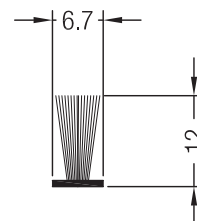
Щеточное уплотнение 6,7 x 12
