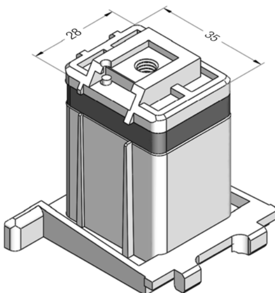
Механический соединитель №2 для импоста 86 BT70
